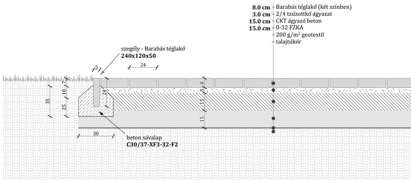
BARABÁS TÉGLAKŐ BURKOLAT / 1:20
